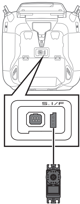
S.BUS/S.BUS2 サーボ
